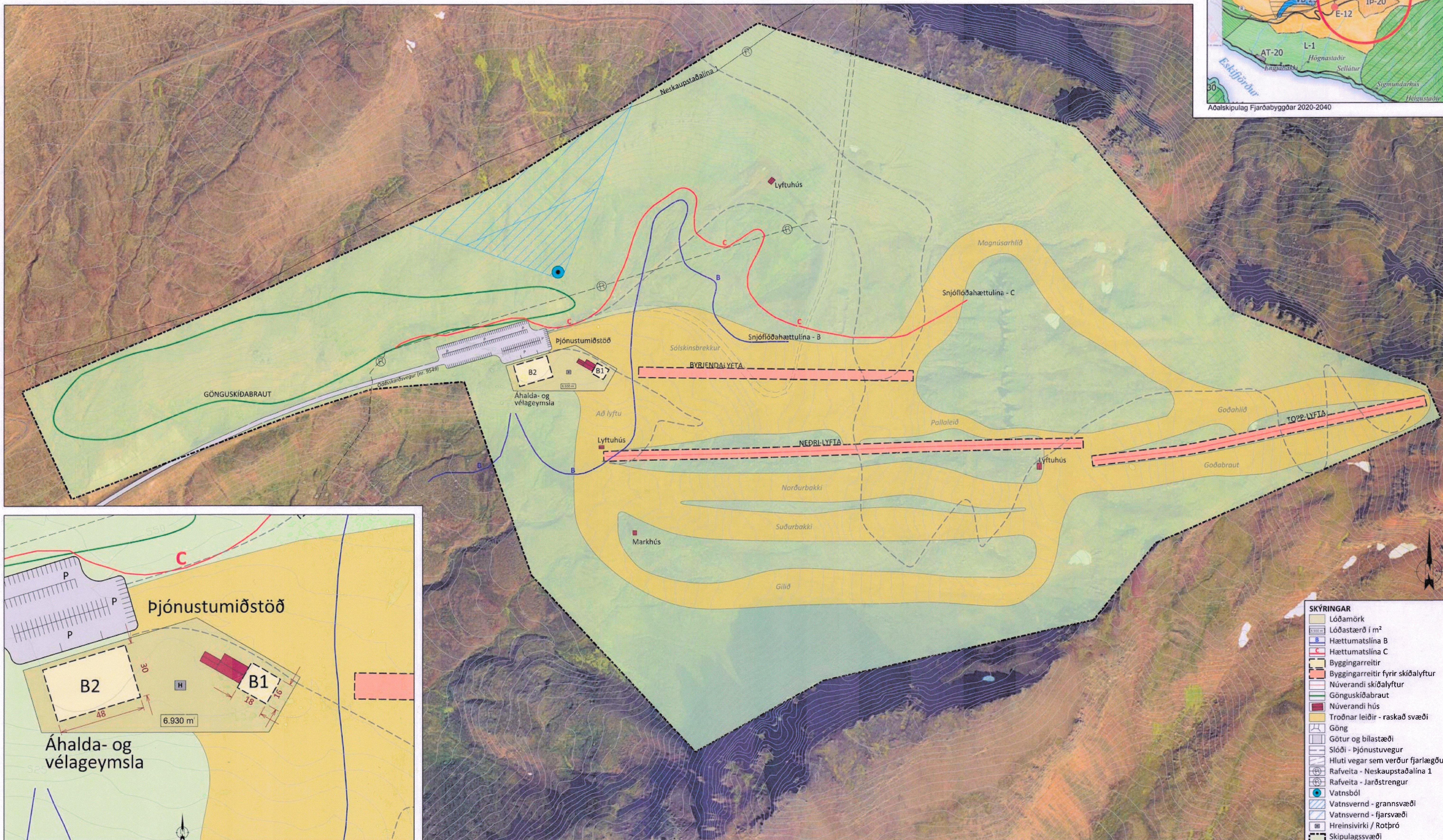
Skýringaruppdráttur fyrir vélageymslu og þjónustumiðstöð í mkv. 1:1000
