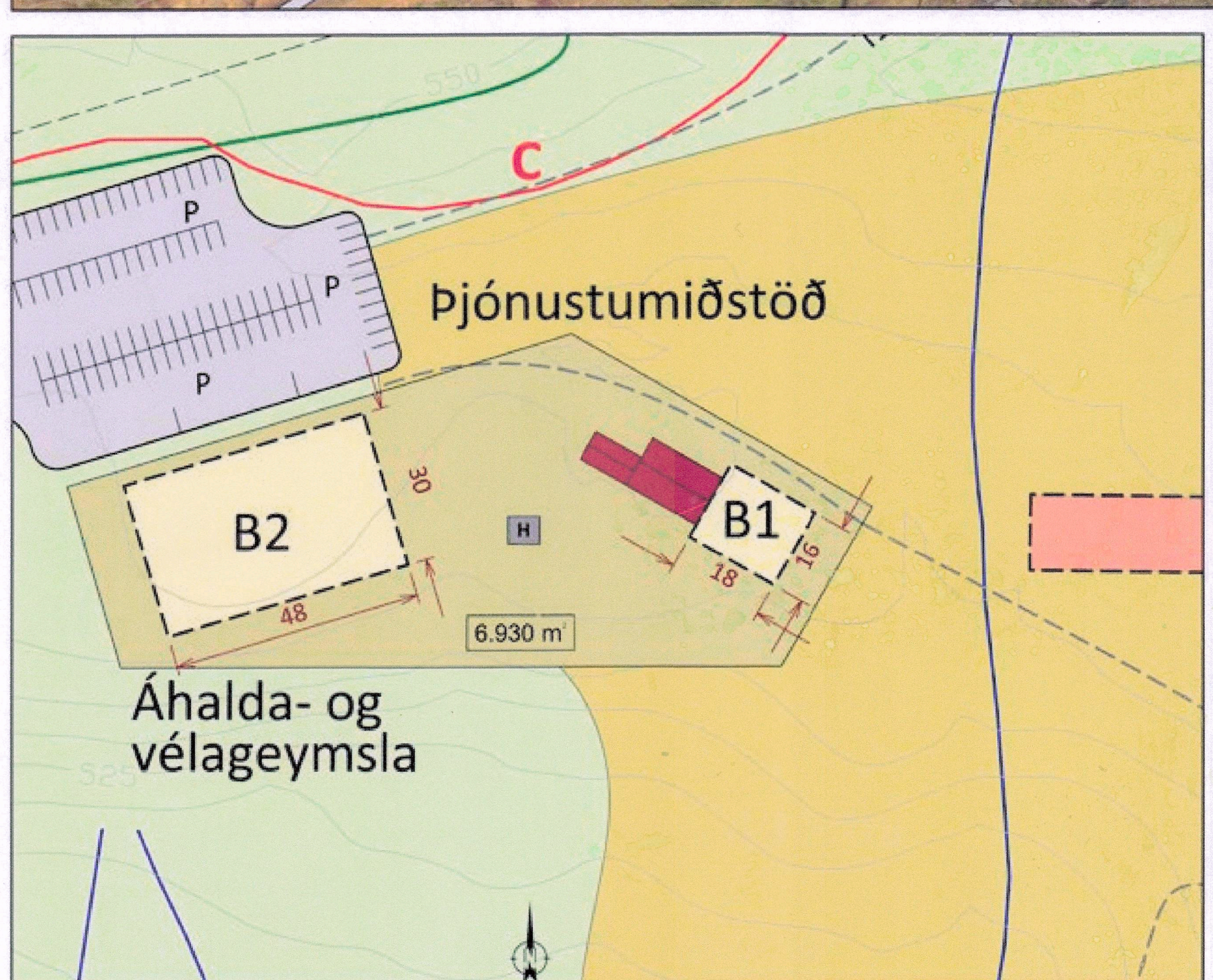
Skýringaruppdráttur fyrir vélageymslu og þjónustumiðstöð í mkv. 1:1000
